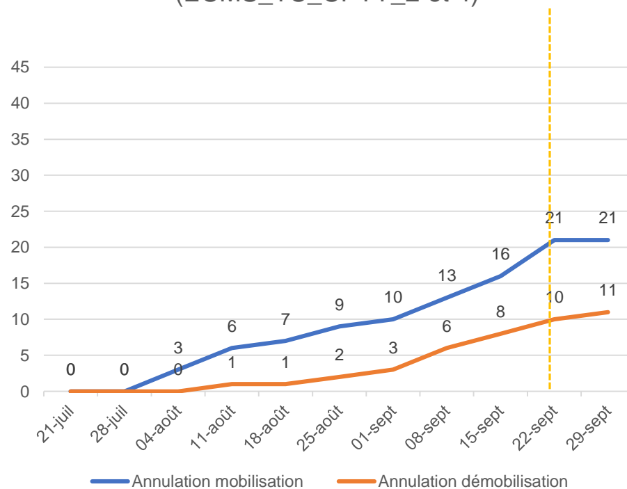
Test d'annulation U2A et A2A (ECMS_TC_CPTY_2 et 4)
